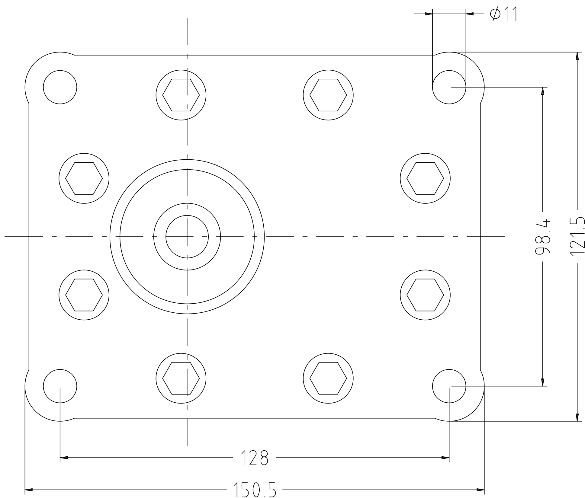
Fissaggio lato motore
